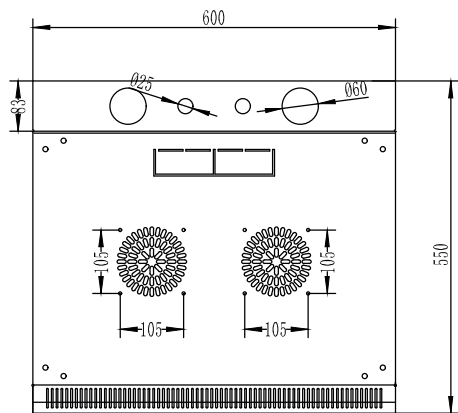
顶部 Top
