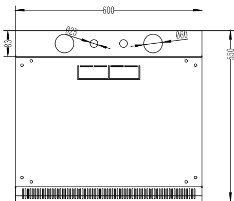
底部 Bottom
