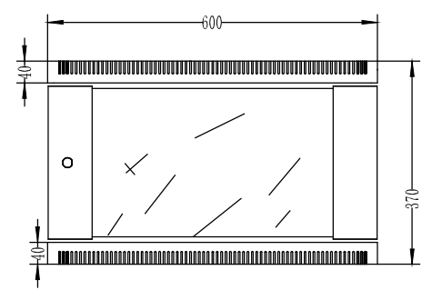
前面 Front
