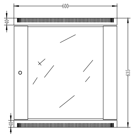
前面 Front
