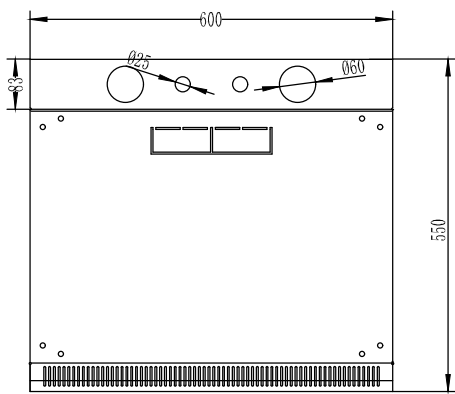
底部 Bottom
