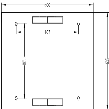
后背 Back
