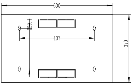
后背 Back
