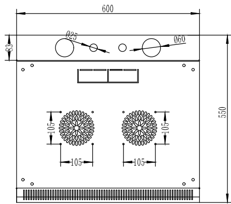
顶部 Top
